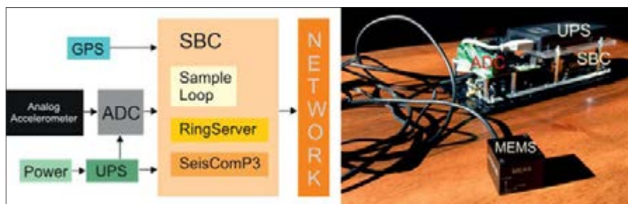
Figura 4 – Schema di lavoro della stazione di monitoraggio (sinistra) e vista interna della stazione assemblata (destra)
