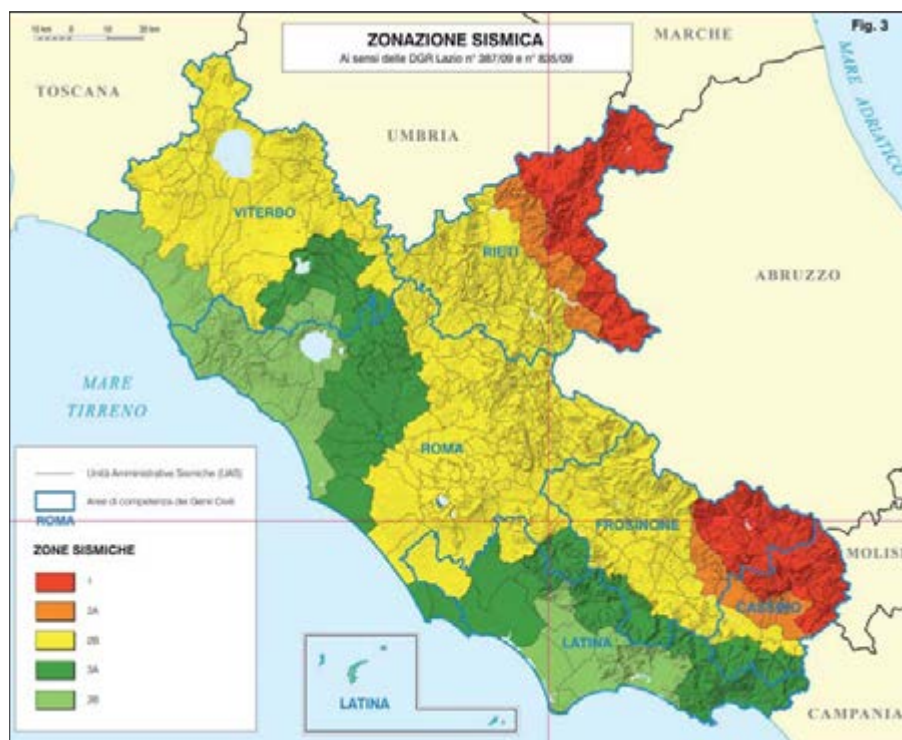
Figura 3 – Zonazione sismica
